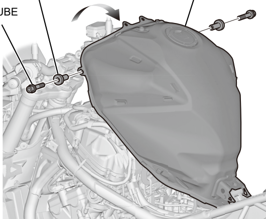
MONTAGEABBILDUNG
