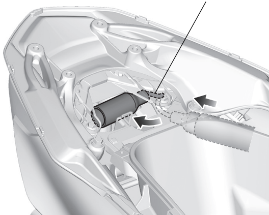
KABELBAUM DES MOTORRADS
